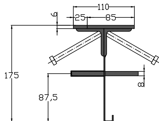
CONECTO 06NE110-5D-T8 h=175 Section
