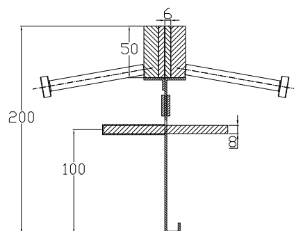
CONECTO SINUS 06NS50-4D-T8 h=200 SECTION
