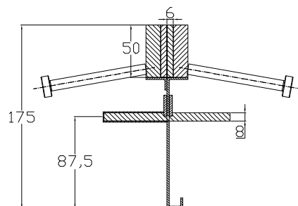
CONECTO SINUS 06NS50-4D-T8 h=175 Section
