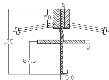
CONECTO SINUS 06NS50-4D-T8 h=175 SECTION
