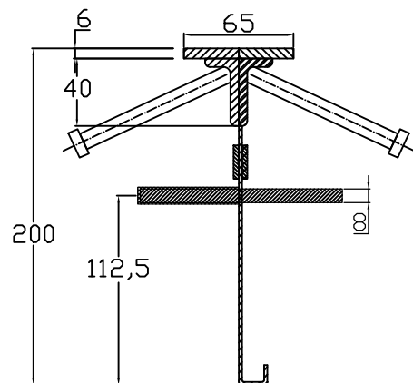
CONECTO SINUS 06NCC65/40x20-5D-T8 h=200 Section
