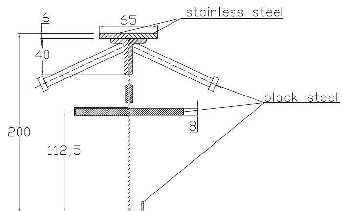
CONECTO SINUS 06NCC65/40x20-5D-T8 h=200 Section
