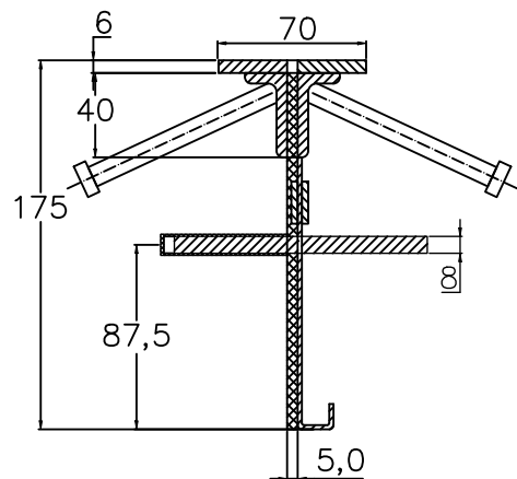
CONECTO SINUS 06NCC65/40x20-5D-T8 h=175 Section
