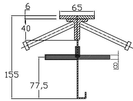
CONECTO SINUS 06NCC65/40x20-5D-T8 h=155 Section
