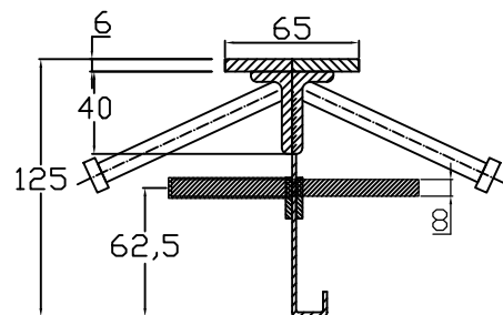
CONECTO SINUS 06NCC65/40x20-5D-T8 h=125 Section
