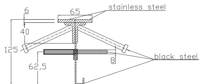
CONECTO SINUS 06NCC65/40x20-5D-T8 h=125 Section
