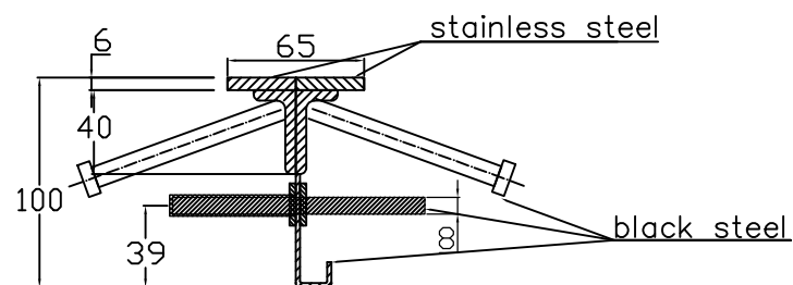
CONECTO SINUS 06NCC65/40x20-5D-T8 h=100 Section
