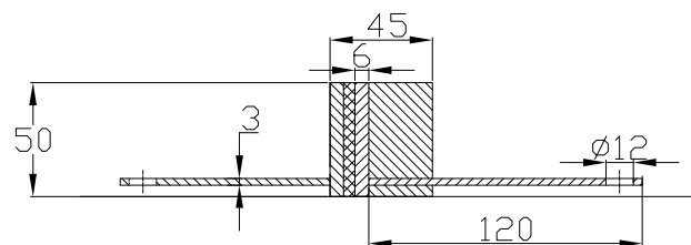
CONECTO SINUS 06NC50-R SECTION
