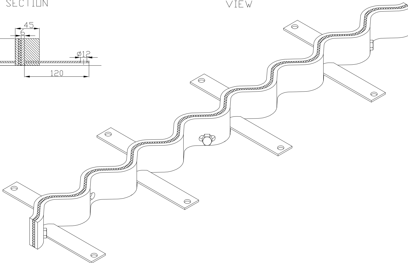
CONECTO SINUS 06NC50-R SECTION
