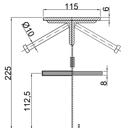
CONECTO SINUS 06NC115-5D-T8 h=225 SECTION
