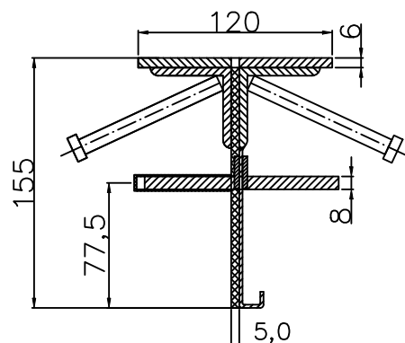
CONECTO SINUS 06NC115-5D-T8 h=155 SECTION
