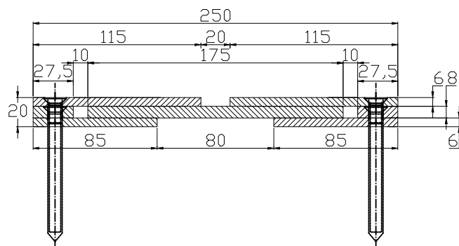
CONECTO ZIGZAG 06NZ250/20-R S80K20 Section
