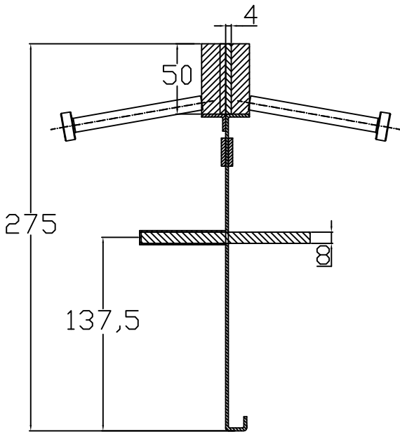
CONECTO SINUS 04NS50-4D-T8 h=275 SECTION
