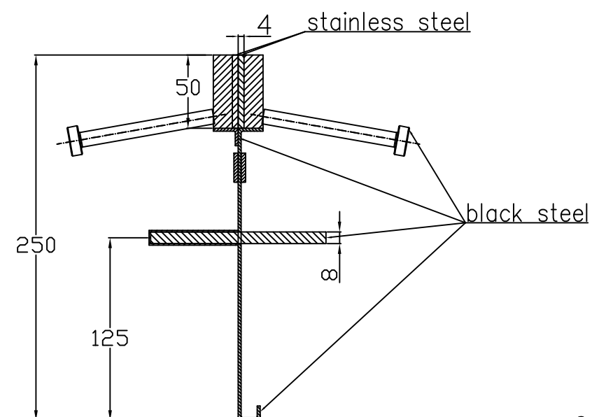
CONECTO SINUS 04NS50-4D-T8 h=250 SECTION
