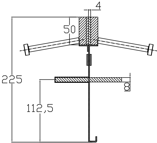
CONECTO SINUS 04NS50-4D-T8 h=225 SECTION
