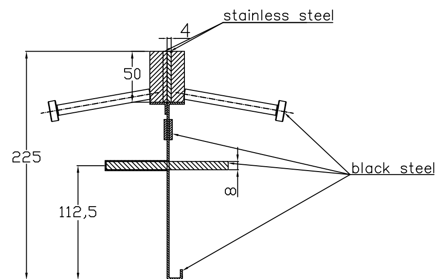
CONECTO SINUS 04NS50-4D-T8 h=225 SECTION
