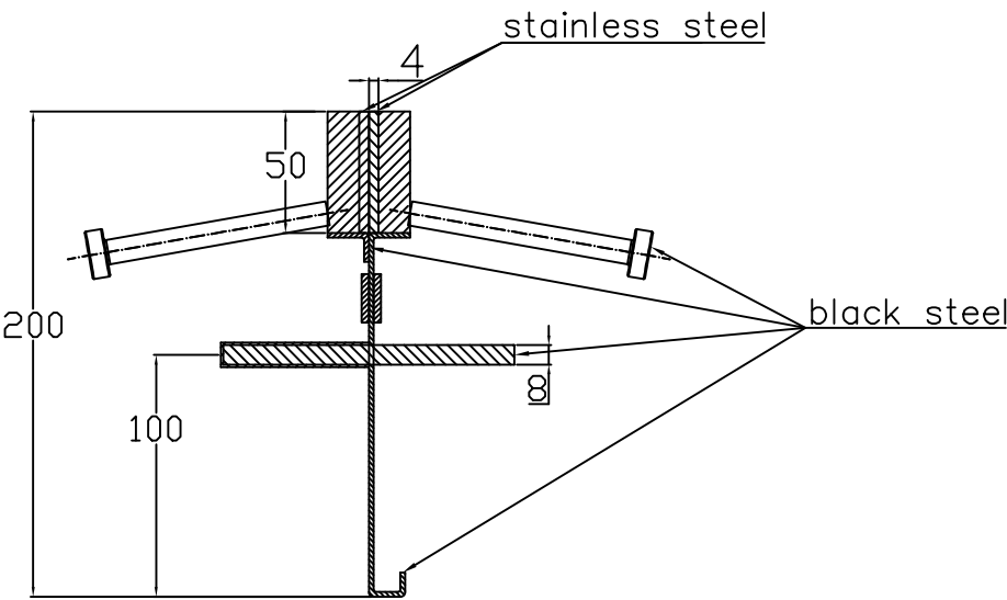
CONECTO SINUS 04NS50-4D-T8 h=200 SECTION
