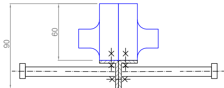
CONECTO SINUS 06NSTW60 h=90 Section SCALE 2:1
