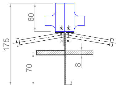
CONECTO SINUS 06NSTW60-5D-T8 h=175 Section
