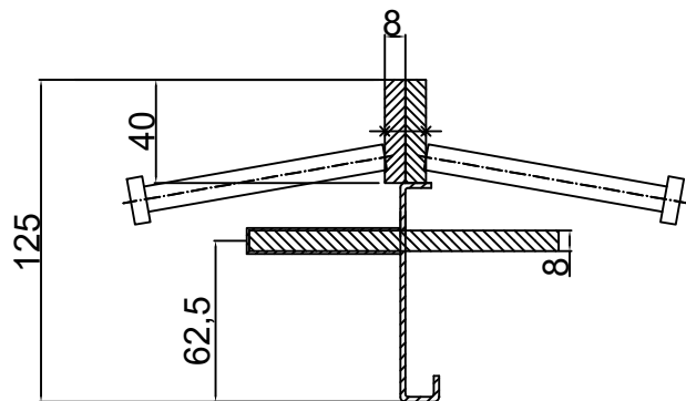
CONECTO DOWEL 08NA40-5D-T8 h=125 Przekrój Skala 2:1
