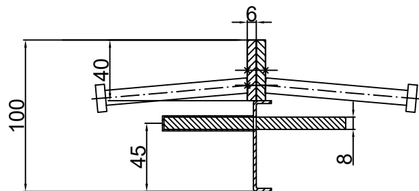
CONECTO DOWEL 06NA40-5D-T8 h=100 Przekrój
