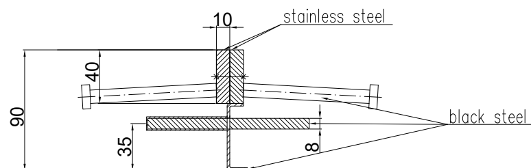
CONECTO DOWEL 10NA40-5D-T8 h=90 SECTION
