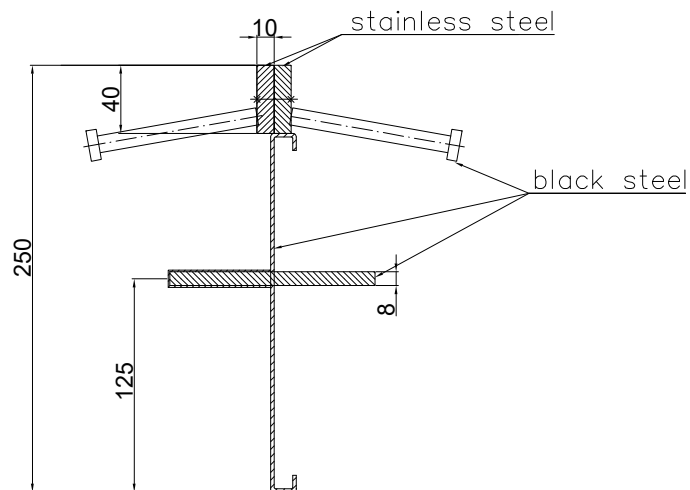
CONECTO DOWEL 10NA40-5D-T8 h=250 SECTION
