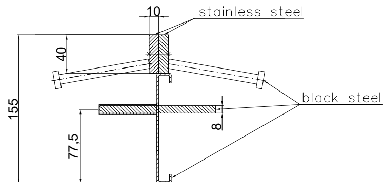
CONECTO DOWEL 10NA40-5D-T8 h=155 SECTION
