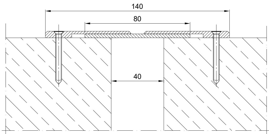
WA 140 SECTION
