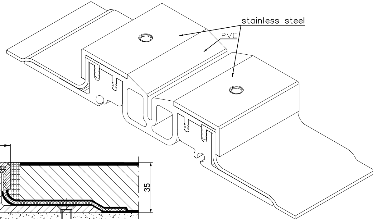
CONECTO GA 63.30.35 L SECTION
