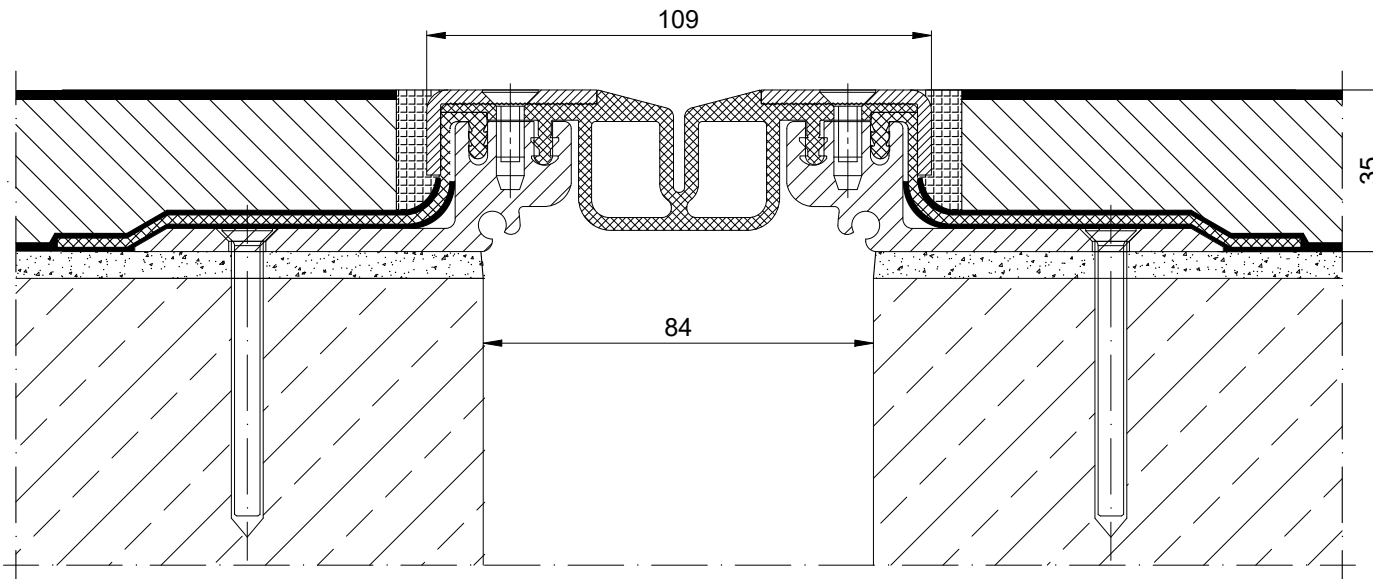
CONECTO GA 63.30.35 L SECTION
