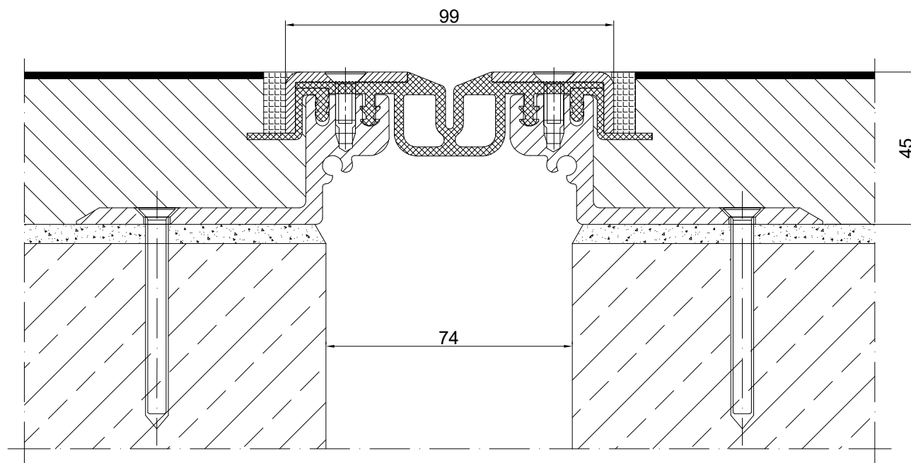
CONECTO GA 50.20.45 S SECTION
