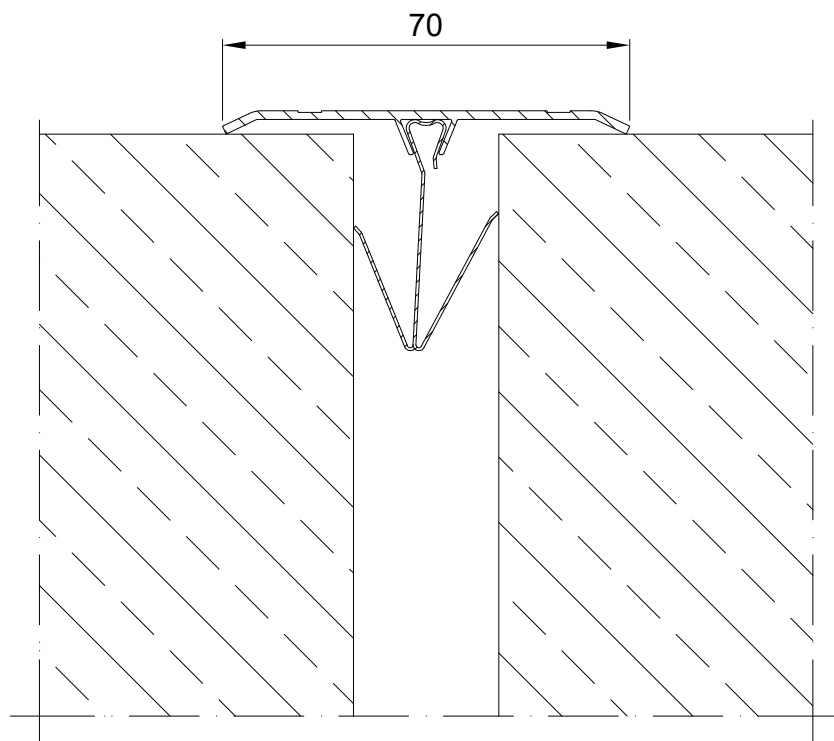
CONECTO JW 70 SECTION
