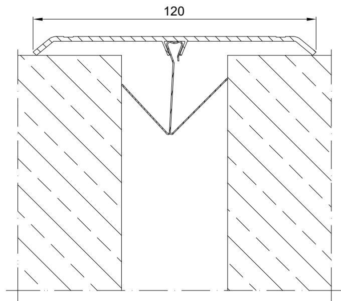
CONECTO JW 120 SECTION
