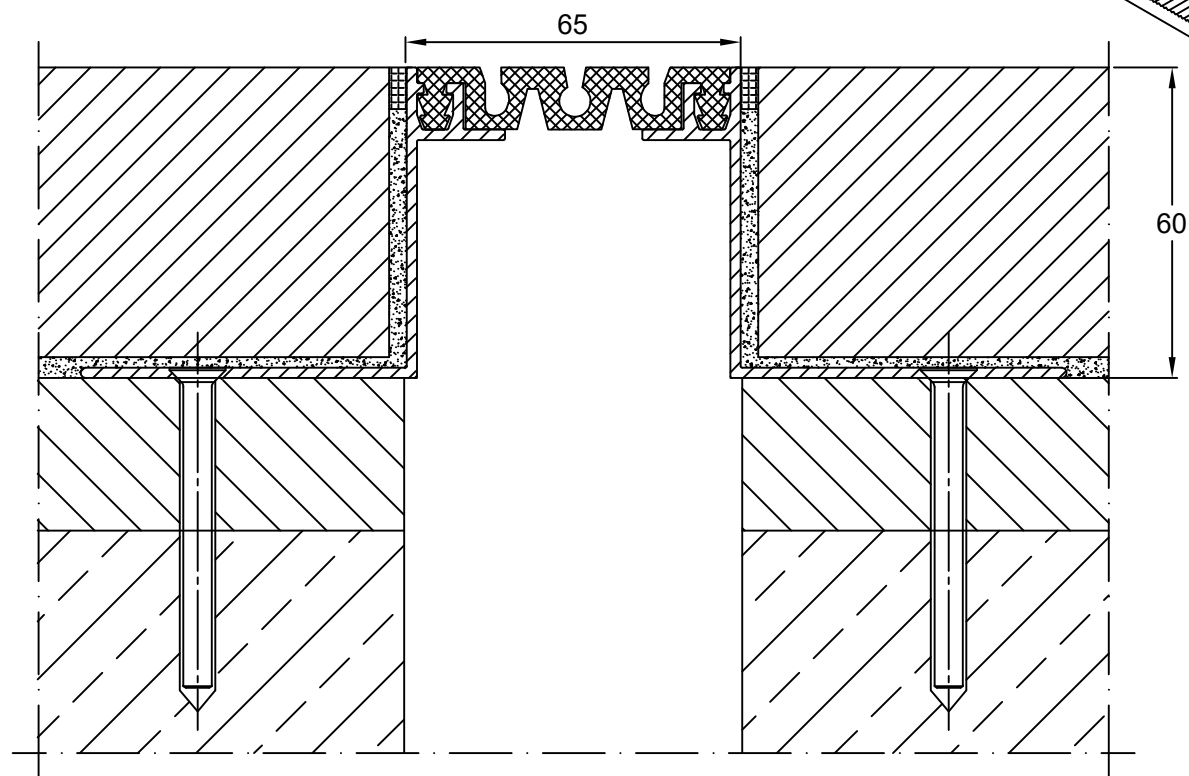
CONECTO EL 65.10.60 SECTION
