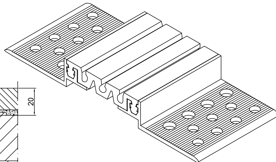
CONECTO EL 65.10.20 VIEW
