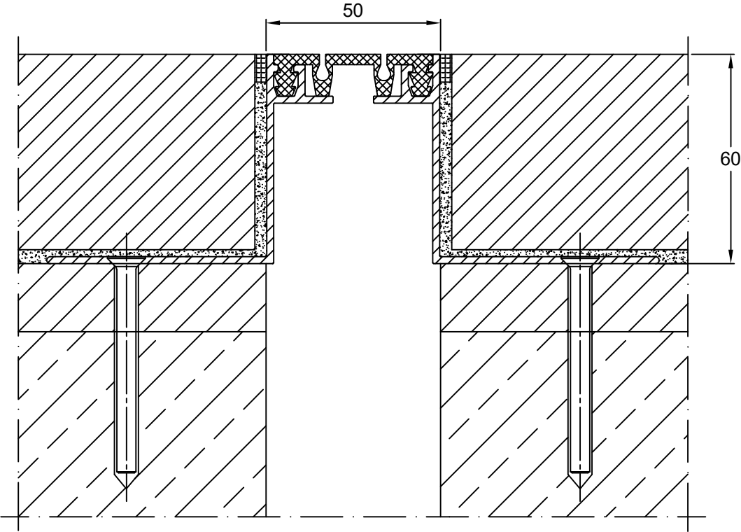
CONECTO EL 50.8.60 SECTION
