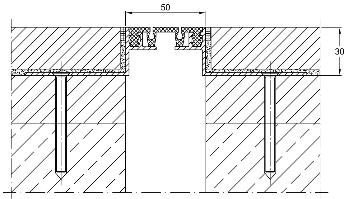
CONECTO EL 50.8.30 SECTION
