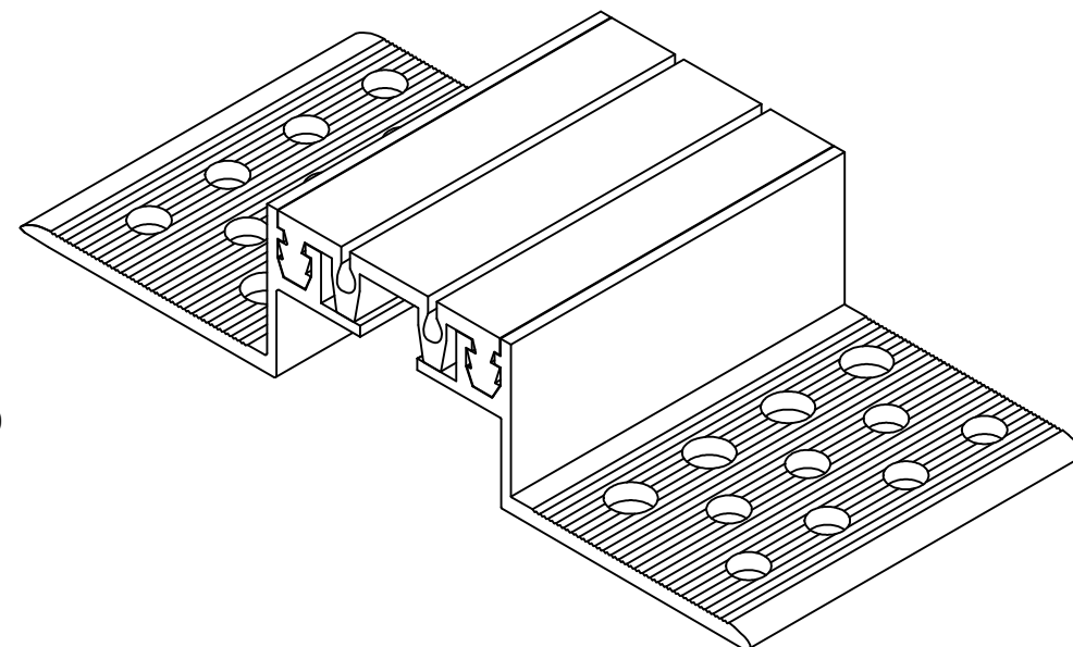
CONECTO EL 50.8.30 VIEW
