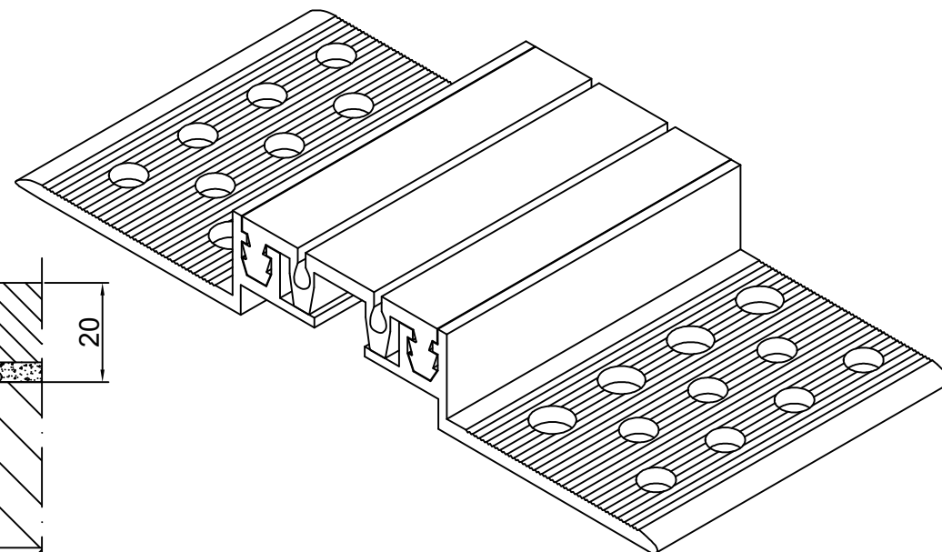
CONECTO EL 50.8.20 VIEW
