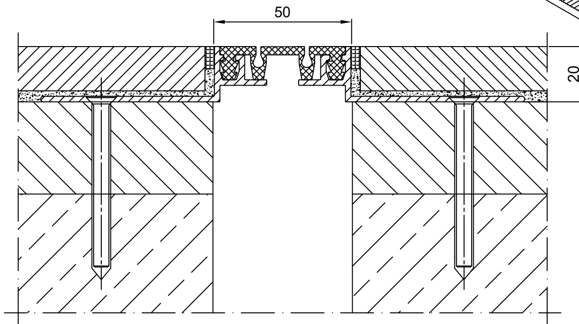
CONECTO EL 50.8.20 SECTION
