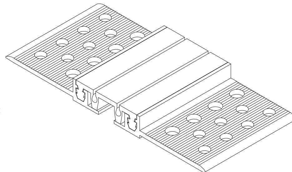
CONECTO EL 50.8.12 VIEW
