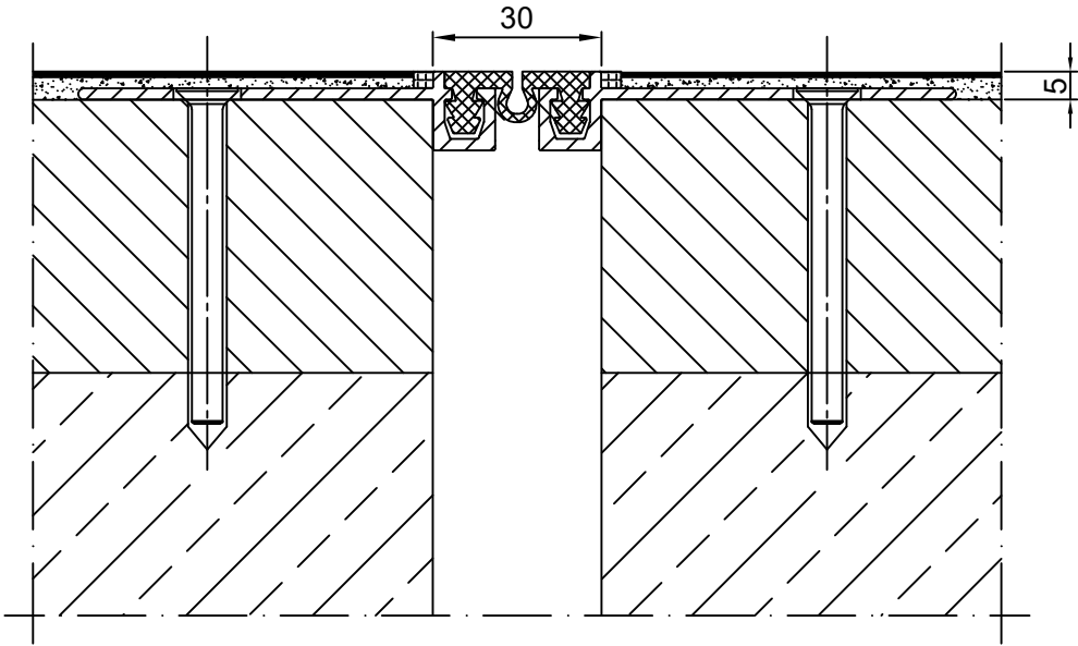
CONECTO EL 30.6.5 SECTION
