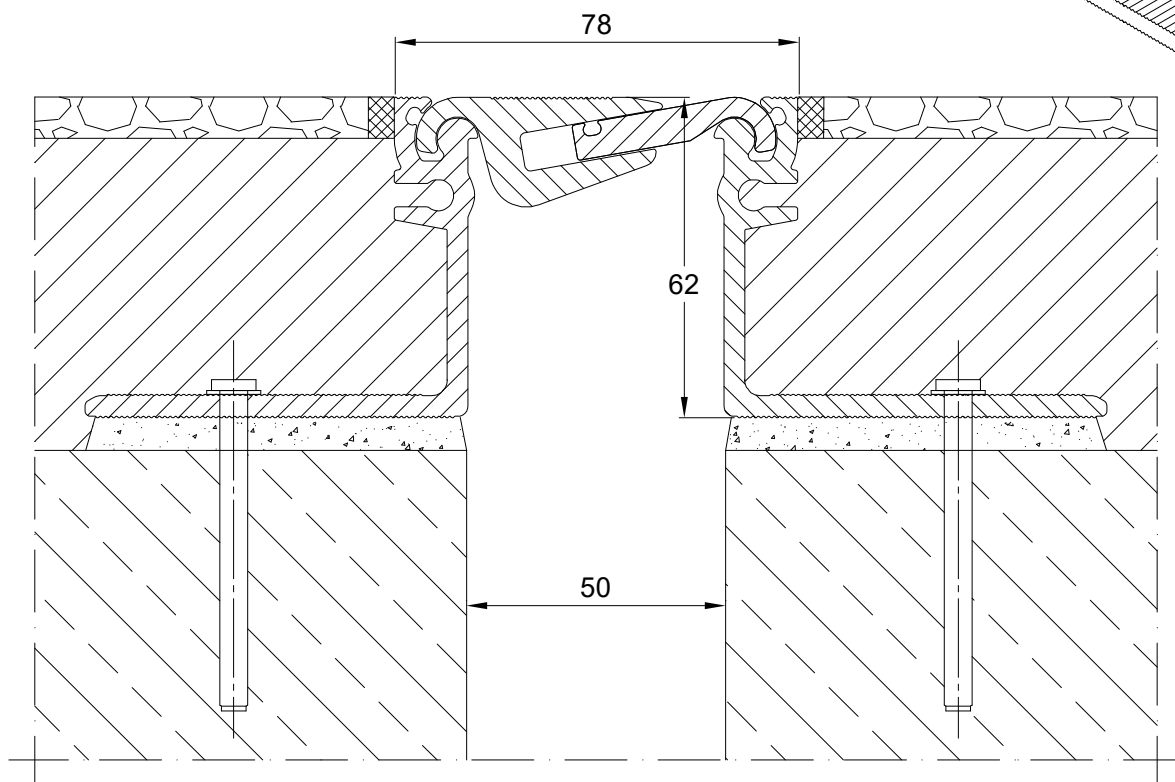
CONECTO AL 78.10.62 SECTION
