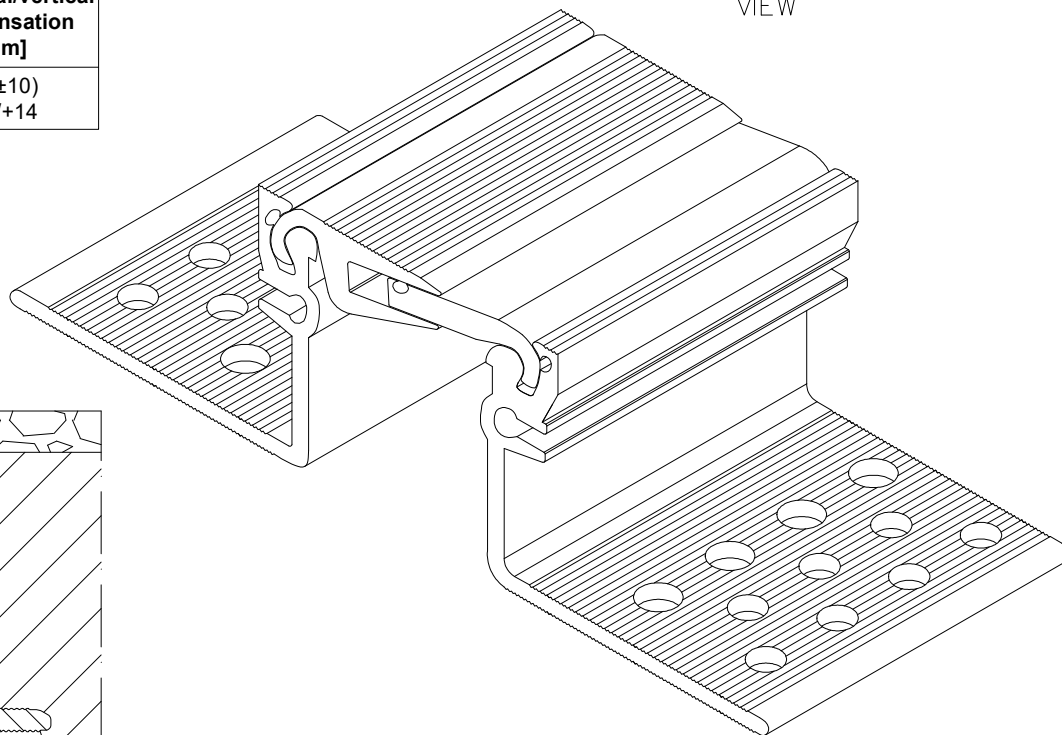
CONECTO AL 78.10.62 VIEW
