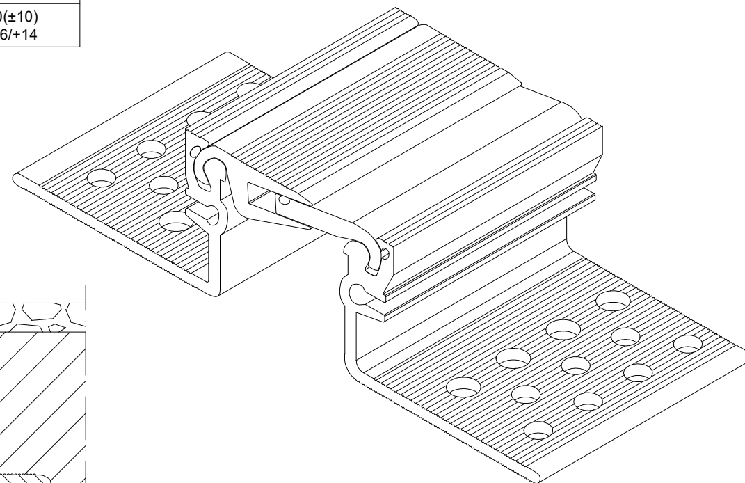
CONECTO AL 78.10.52 VIEW
