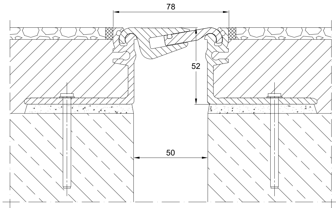
CONECTO AL 78.10.52 SECTION
