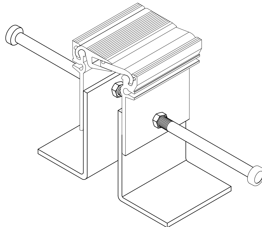
CONECTO AL 78.10.120& VIEW
