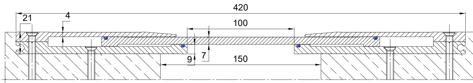
Conecto AL 420/21 Section SCALE 1:1,75
