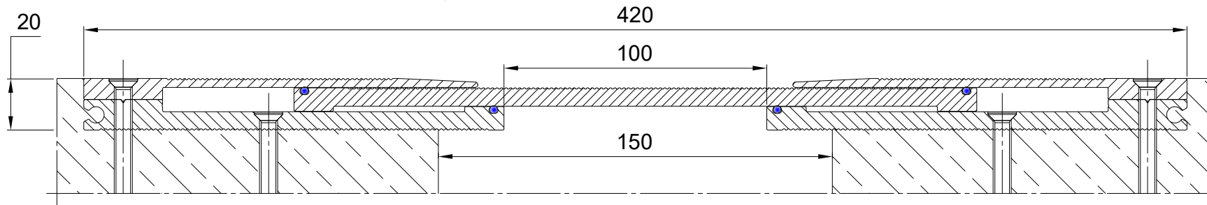
Conecto AL 420 SECTION SCALE 1:1,75
