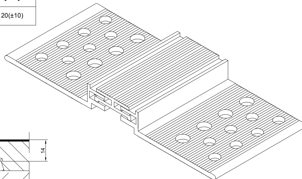
CONECTO AL 38.10.14 View
