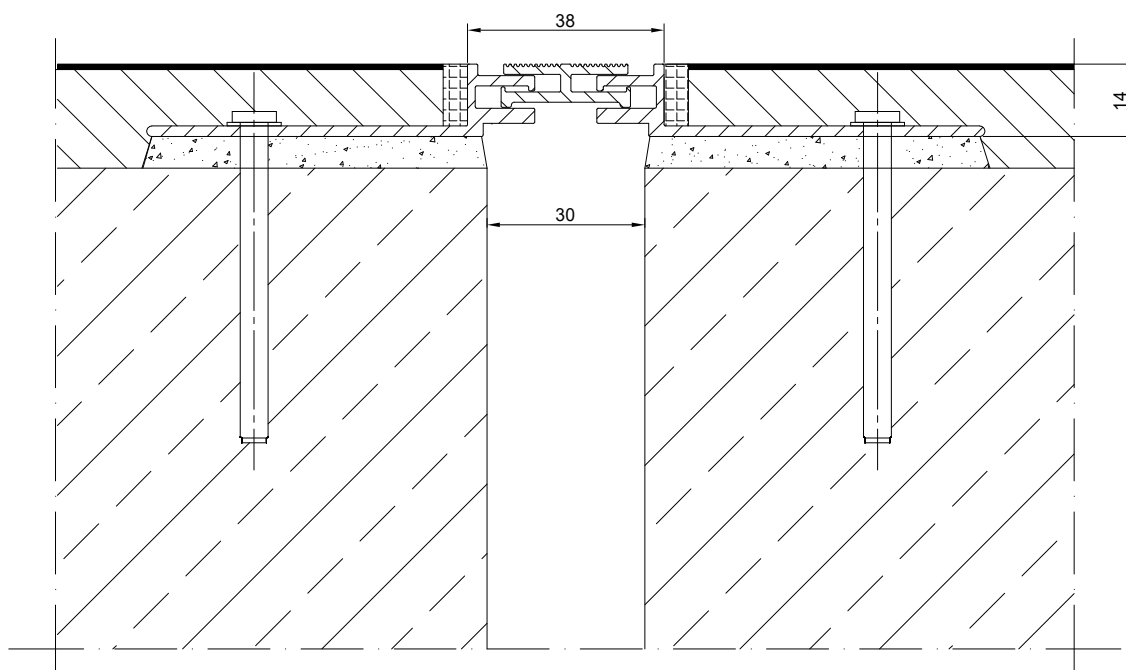
CONECTO AL 38.10.14 SECTION
