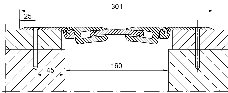
CONECTO AL 165.30.N SECTION SCALE 1:2
