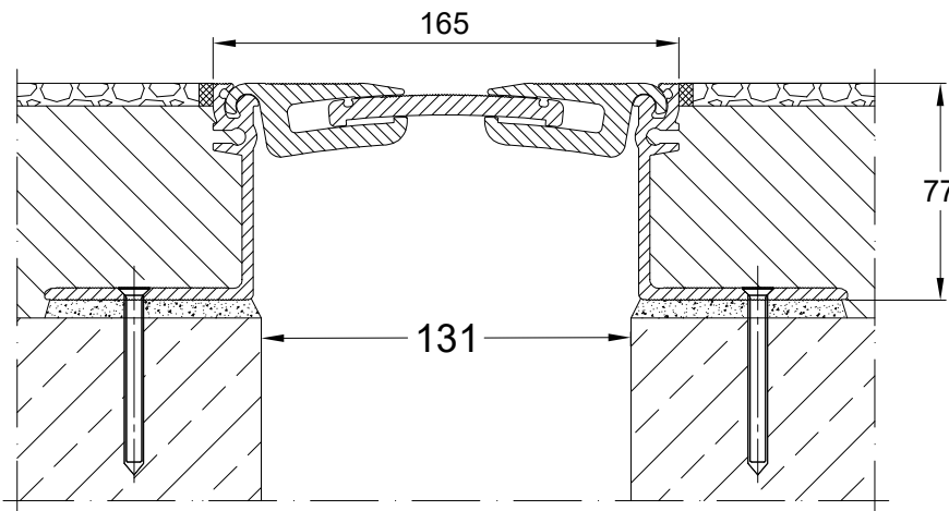
CONECTO AL 165.30.77 SECTION SCALE 1:2
