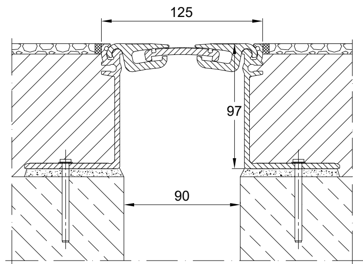
CONECTO AL 125.20.97 SECTION SCALE 1:2
