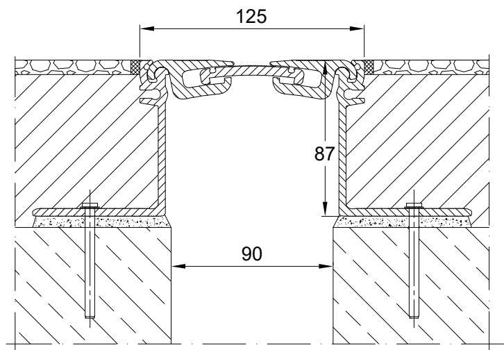
CONECTO AL 125.20.87 SECTION SCALE 1:2
